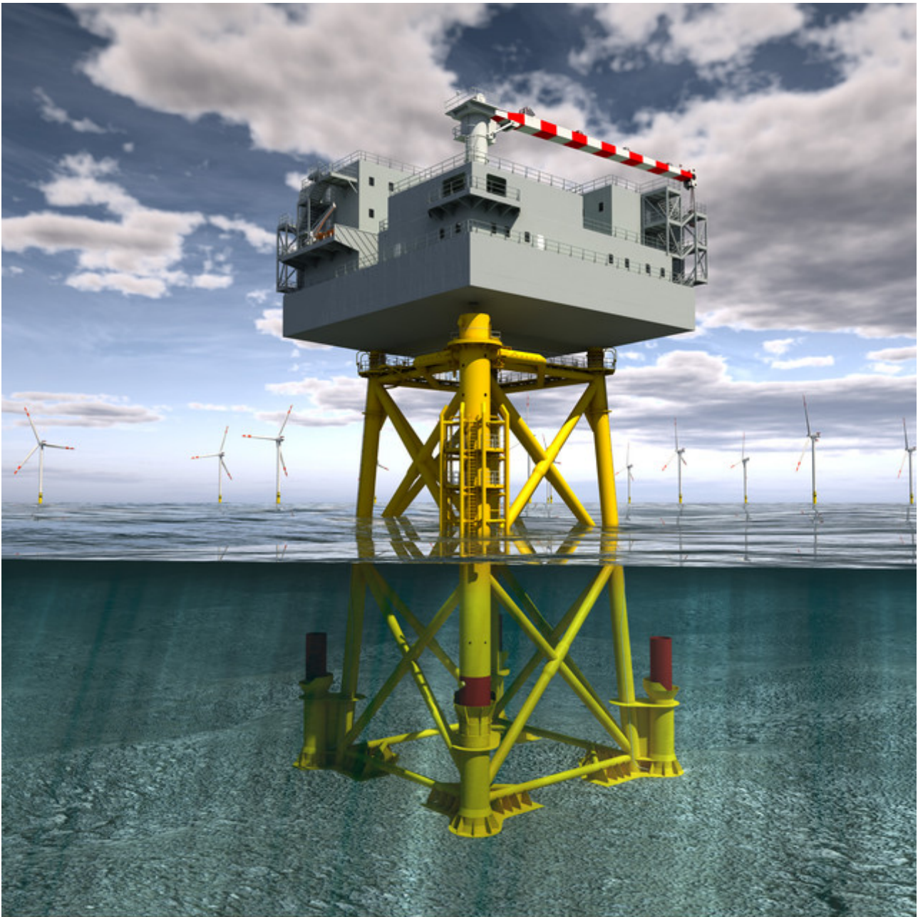
Wohnplattform Wasserschnitt
